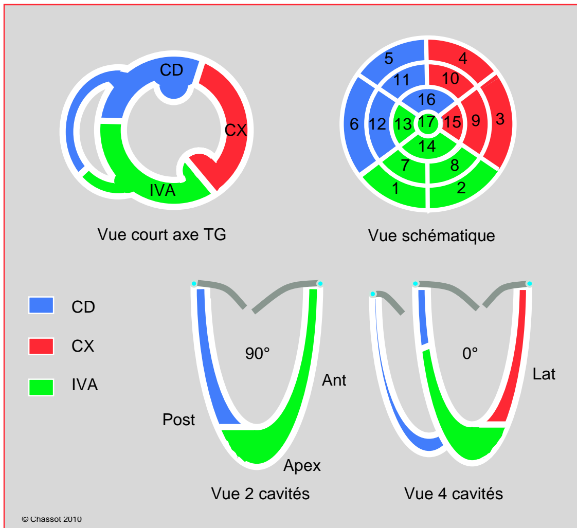
Figure 27.3 : Territoires coronariens en vue court axe transgastrique (TG), en vues 2 cavités et 4 cavités rétrocardiaques, et en vue schématique. Cette dernière est une projection circulaire centrée sur l'apex de la vascularisation des différents segments. CD : artère coronaire droite. CX : artère circonflexe. IVA : artère interventriculaire antérieure. Les segments 13, 15 et 17 peuvent être vascularisés par la CD (interventriculaire postérieure) ou l'IVA (interventriculaire antérieure). Le segment 14 peut être vascularisé par l'IVA ou la CX, et le segment 16 par la CX ou la CD.
